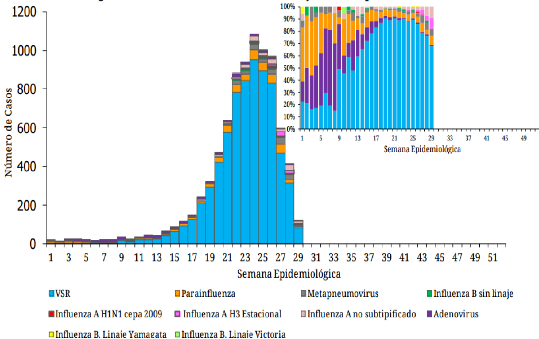
Figura 4 – Distribución de virus respiratorios en vigilancia por Semana epidemiológica. SE1 a SE 29 de 2015. Argentina. Muestras analizadas (N)= 30154 y Muestras positivas (n)=8431
