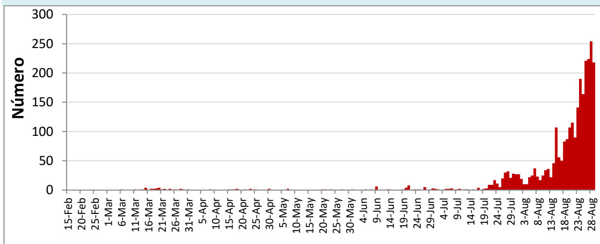
Fig. 5. Curva epidémica de casos confirmados de COVID-19 según fecha de inicio de síntomas. Provincia de Tucumán, hasta agosto de 2020.
