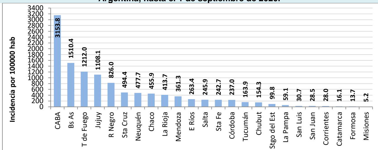
Fig. 2. Incidencia acumulada de COVID-19 (por 100.000 hab.) según jurisdicciones de Argentina, hasta el 1 de septiembre de 2020.
