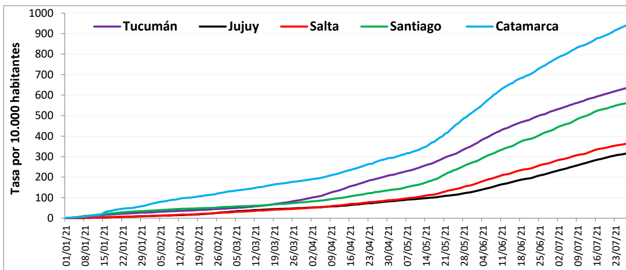
Fig. 3. Curva de Tasas diarias acumuladas de COVID-19 por 10.000 habitantes en provincias del NOA. Argentina – Enero hasta el 27/07/2021
